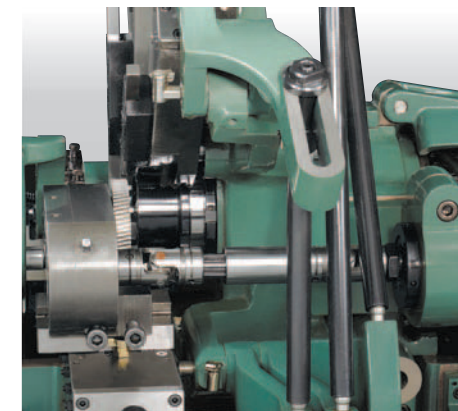
銑牙座
