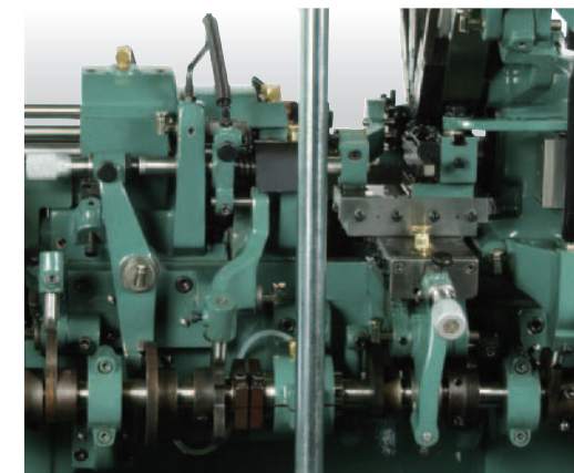
凸輪組
